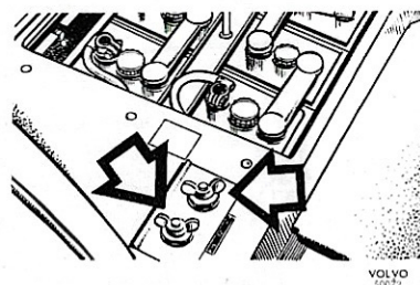
Bild 8. Hjälpstartanslutning
