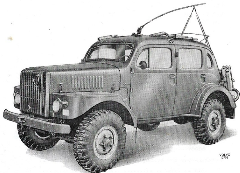
Bild 1. Raptgbil 915 från vänster
