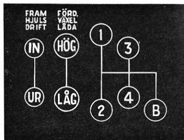
Bild 6. Manöverspakarnas lägen
