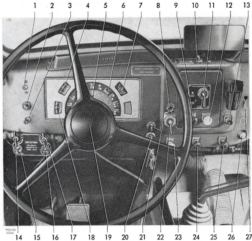
Bild 3. Manöverorgan och instrument
